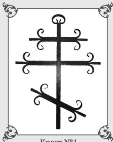
Крест №1 Труба профильная 40x20, 15x15 Высота - 2,1 м
